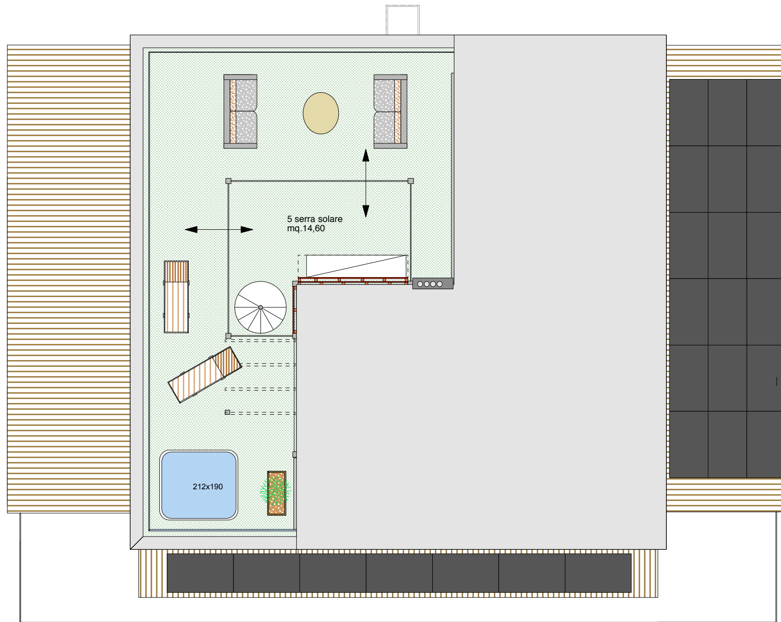
PIANTA PIANO COPERTURA arredi scala 1/100 18.04.23
